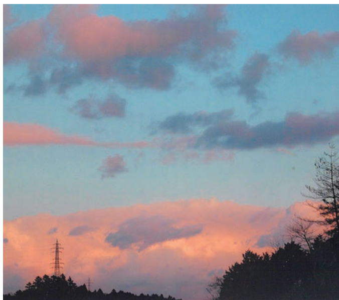
下奥の左右に広がるペール雲（積雲）、中段左右に伸びた筋雲（巻雲）、上部に散在する羊雲（高積雲）
